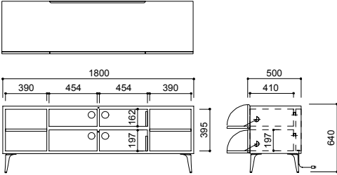
CA-001 Type-A W1800・D500・H640 (AL・H660) (図はアルミ脚)
