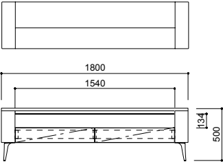
CA-016W-HC W1800・D450・H500
