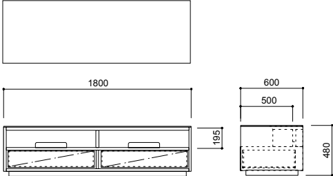
CA-017-HM W1800・D600、450・H480
