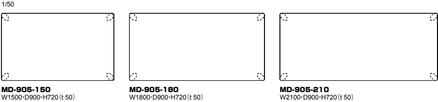
MD-905-150 W1500・D900・H720(t.50)
