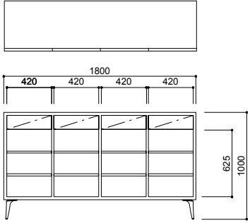
CA-012L W1800・D470・H1010 (W・H1030) (図はアルミ脚)
