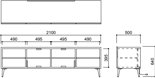
CA-002 Type-B W2100・D500・H640 (AL・H660) (図はアルミ脚)
