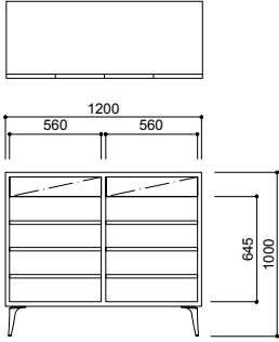
CA-012M W1200・D470・H1010 (W・H1030) (図はアルミ脚)
