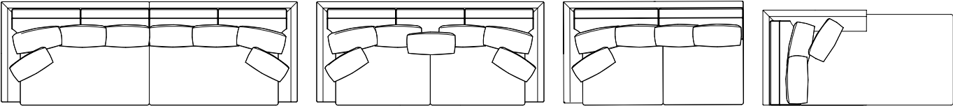
NC-009-4P (2PR+2PL) W2800 (W1400 × W1400) × D980 × H800 (SH400) AH650 (Lクッション×6 Sクッション×2) NC-009-3P W2150 × D980 × H800 (SH400) AH650 (Lクッション×5 Sクッション×2) NC-009-2LR / 2LL W1700 × D880 × H800 (SH400) AH650 (Lクッション×4 Sクッション×1) NC-009-CLL/CLR W900 × D1800 × H800 (SH400) AH650 (Lクッション×2 Sクッション×1)
