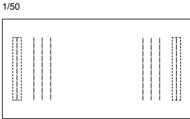
MD-107L-180 W1800・D950・H650(t 50)
