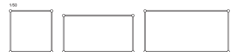
AD-006 (90) W935-D935-H700 (t 80) AD-006 (150) W1535-D835-H700 (t 80) AD-006 (180) W1835-D935-H700 (t 80)
