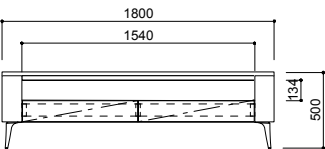
CA-016W-HC W1800・D450・H500
