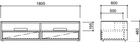
CA-017-HO W1800・D600、450・H480
