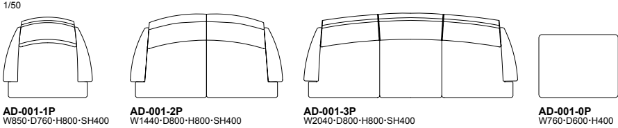
AD-001-1P W850・D760・H800・SH400
