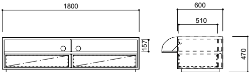
CA-017-HM W1800・D600、450・H470
