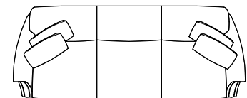
NC-016-3P W2150 × D880 × H850 (SH410)AH600 (Sクッション×4)
