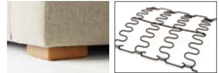
▲NC-046 木製レッグ NC-046 ソファの脚部には、木製脚が取り付けられています。 ▲ウェーブスプリング ウェーブスプリングが座フレーム内に使用されており、ホールド感のある座り心地が得られます。
